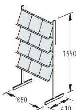
P-12L 4 estantes para 12 folletos DIN A4
