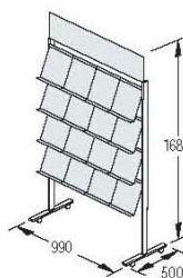
P-16T 4 estantes para 16 folletos DIN A4 + panel superior
