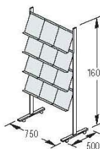
P-12 4 estantes para 12 folletos DIN A4
