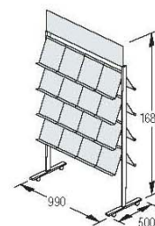
P-32T 8 estantes para 32 folletos DIN A4 + panel superior
