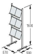
P-6 3 estantes para 6 folletos DIN A4
