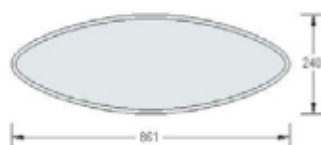
VA 7501 Cubierta VA 7500, madera negra, 10 mm
