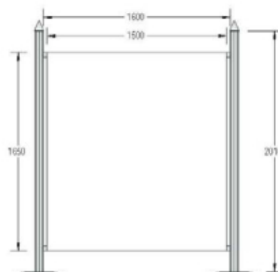
M 1350 Kit banderola central 2 columnas, Ø 80 mm, con bases y conos 2 travesaños long. 1600 mm con grapas
