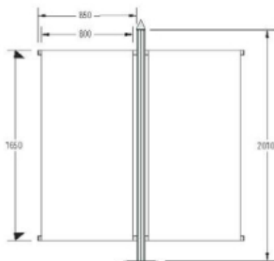
M 1352 Kit banderola a dos lados 1 columna, Ø 80 mm, con base y cono 4 travesaños long. 850 mm con grapa y tapeta
