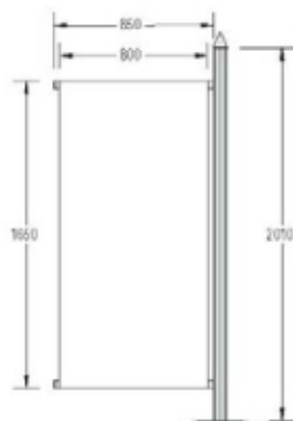
M 1351 Kit banderola a un solo lado 1 columna, Ø 80 mm, con base y cono 2 travesaños long. 850 mm con grapa y tapeta
