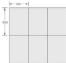
VA 1680 Módulo de 6 marcos
