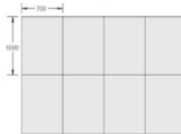
VA 1880 Módulo de 8 marcos
